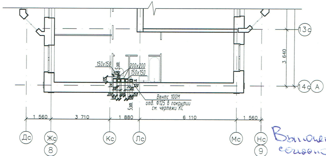
Фрагмент плана 5 этажа в осях 9-8, А.
