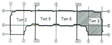
Схема блокировки
