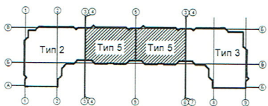
Схема блокировки
