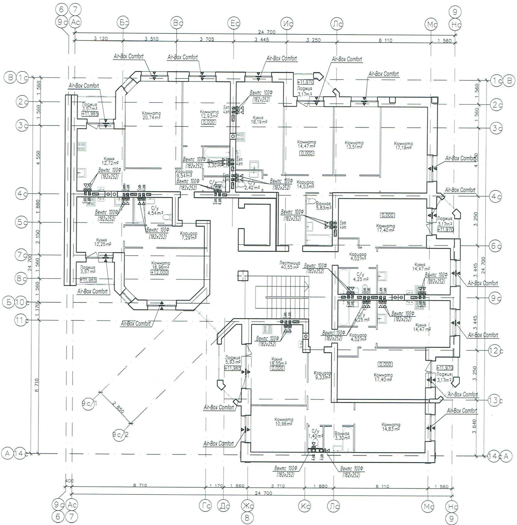
Фрагмент плана 5 этажа в осях 9-8, А.
